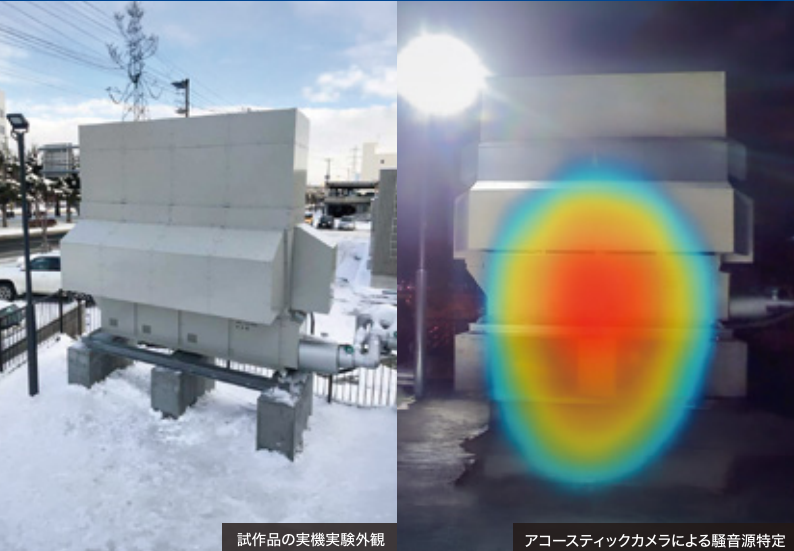
試作品の実機実験外観
