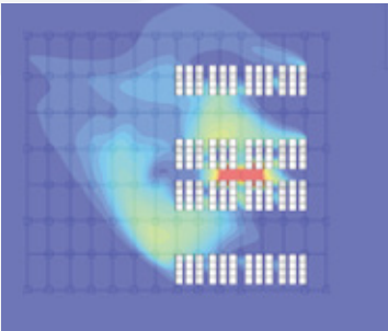
気流解析イメージ
