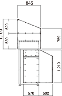
側面図(各型名共通)
