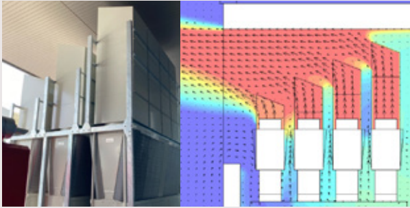
特注品にも柔軟に対応可能 材質変更や形状変更など、様々な特注品の製作実績があります。気流・騒音解析も必要に応じ行いながら現場に最適な製品をご提案・製作します。
