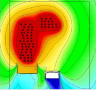
騒音解析イメージ 隣地境界線上での騒音値を解析、基準値以下となるかを確認し対策を検討します。
