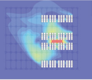
気流解析イメージ 室外機周囲の気流を解析、ショートサーキットによる吸込空気温度上昇を確認し、改善案を検討します。
