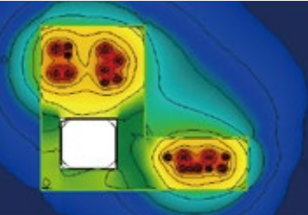
▼ 遮音パネル+防音ダクト設置
