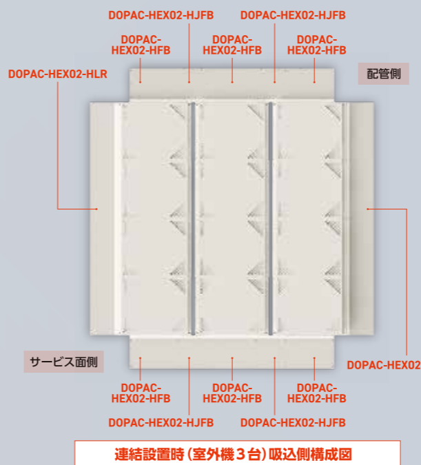
連結設置時(室外機3台)吸込側構成図
