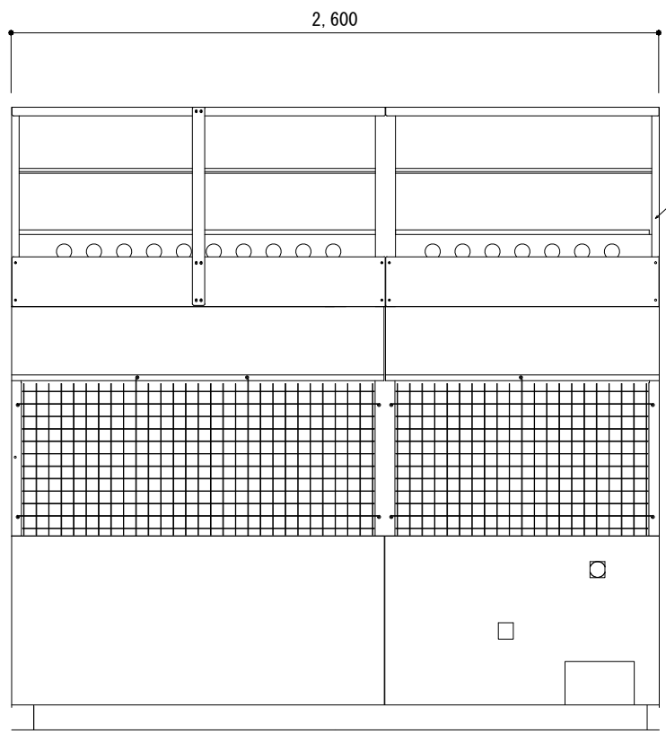
正面図
