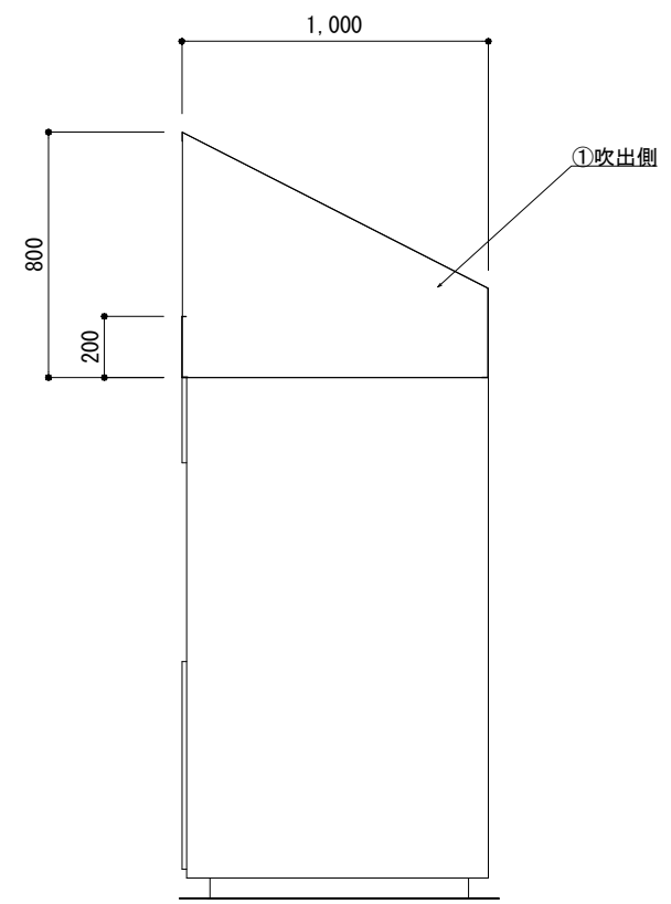
側面図
