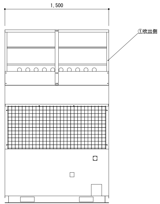
正面図
