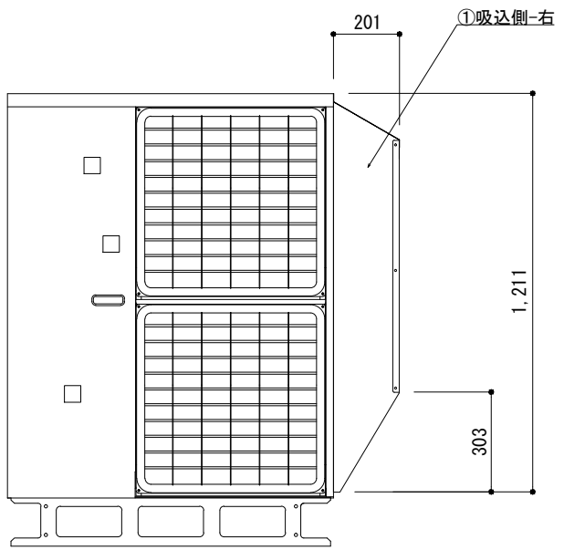
正面図
