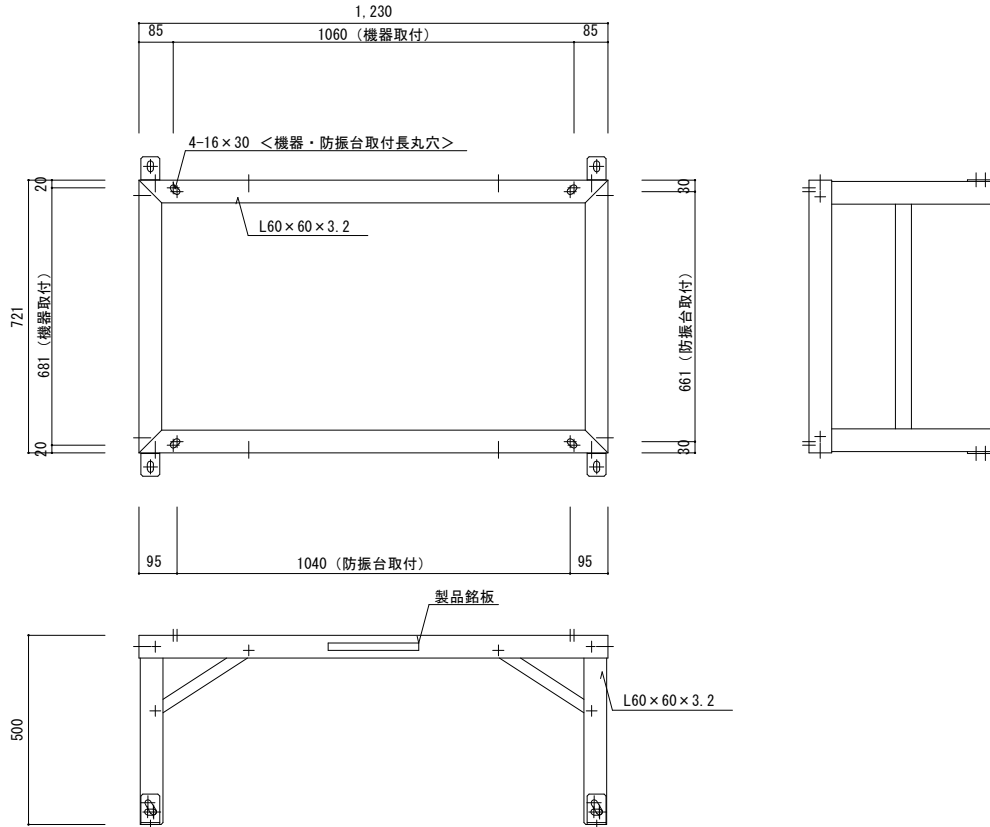
<外形寸法図> S=1/20
