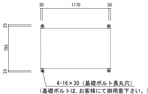
<基礎ボルト位置> S=1/40
