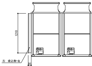
背面図
