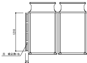
背面図
