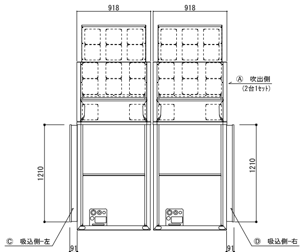
背面図
