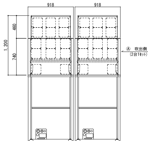
背面図
