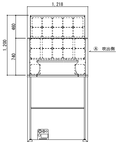
背面図
