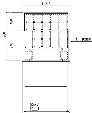
背面図
