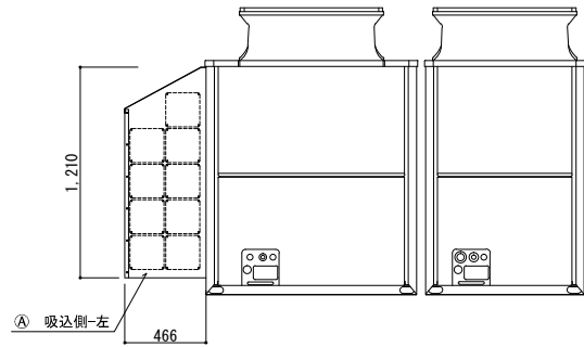
背面図
