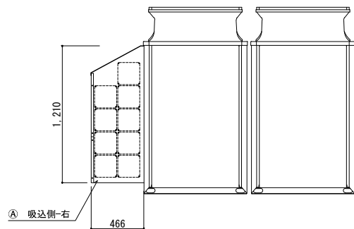
背面図
