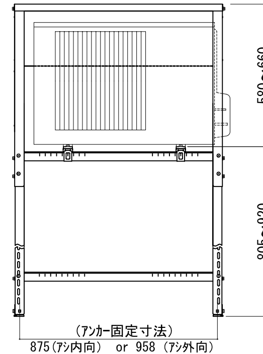
正面図
