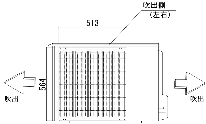
正面図
