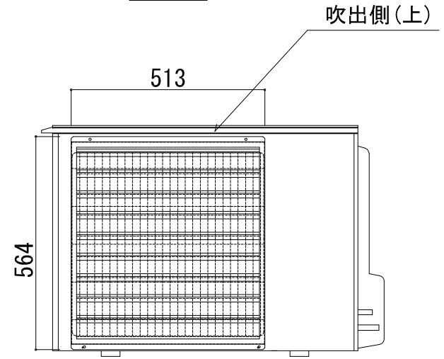
正面図
