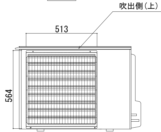
正面図
