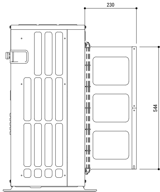
側面図
