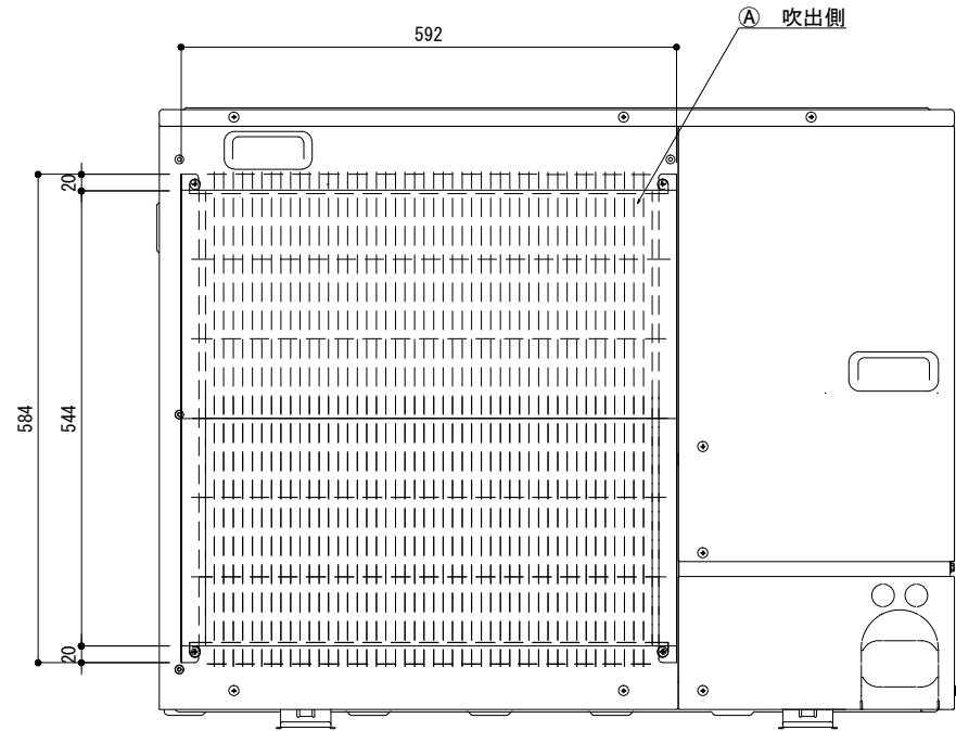
正面図
