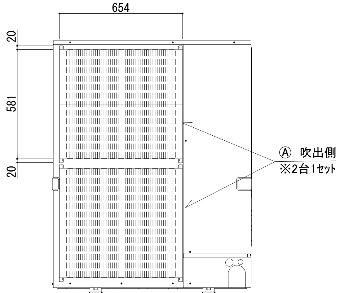
正面図
