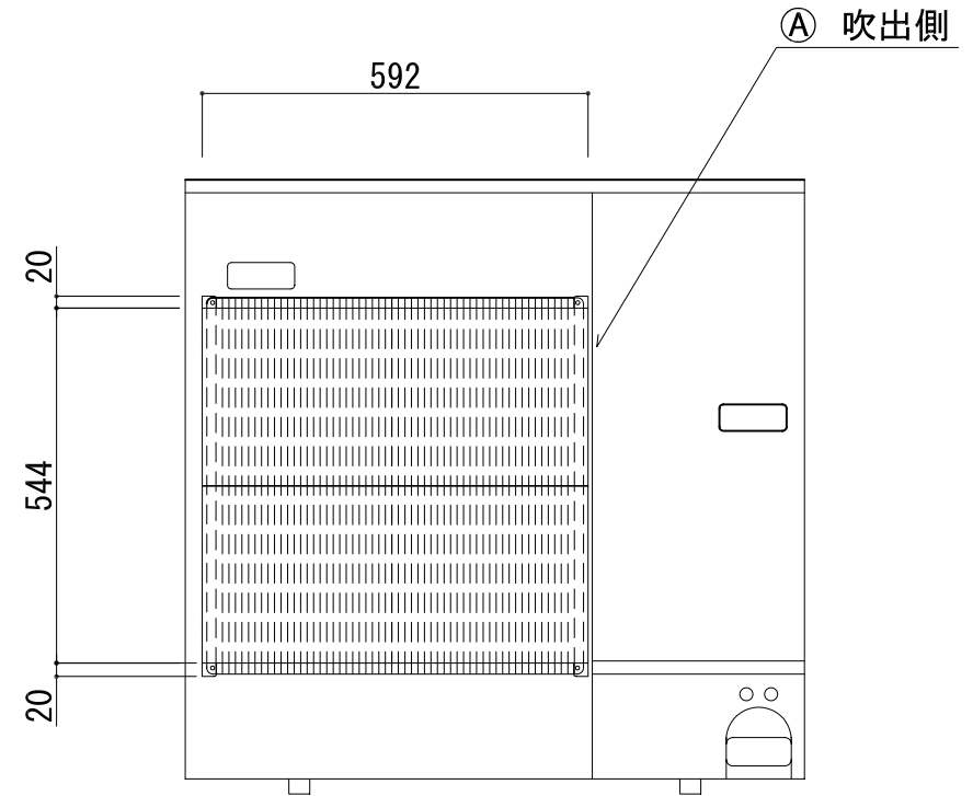
正面図
