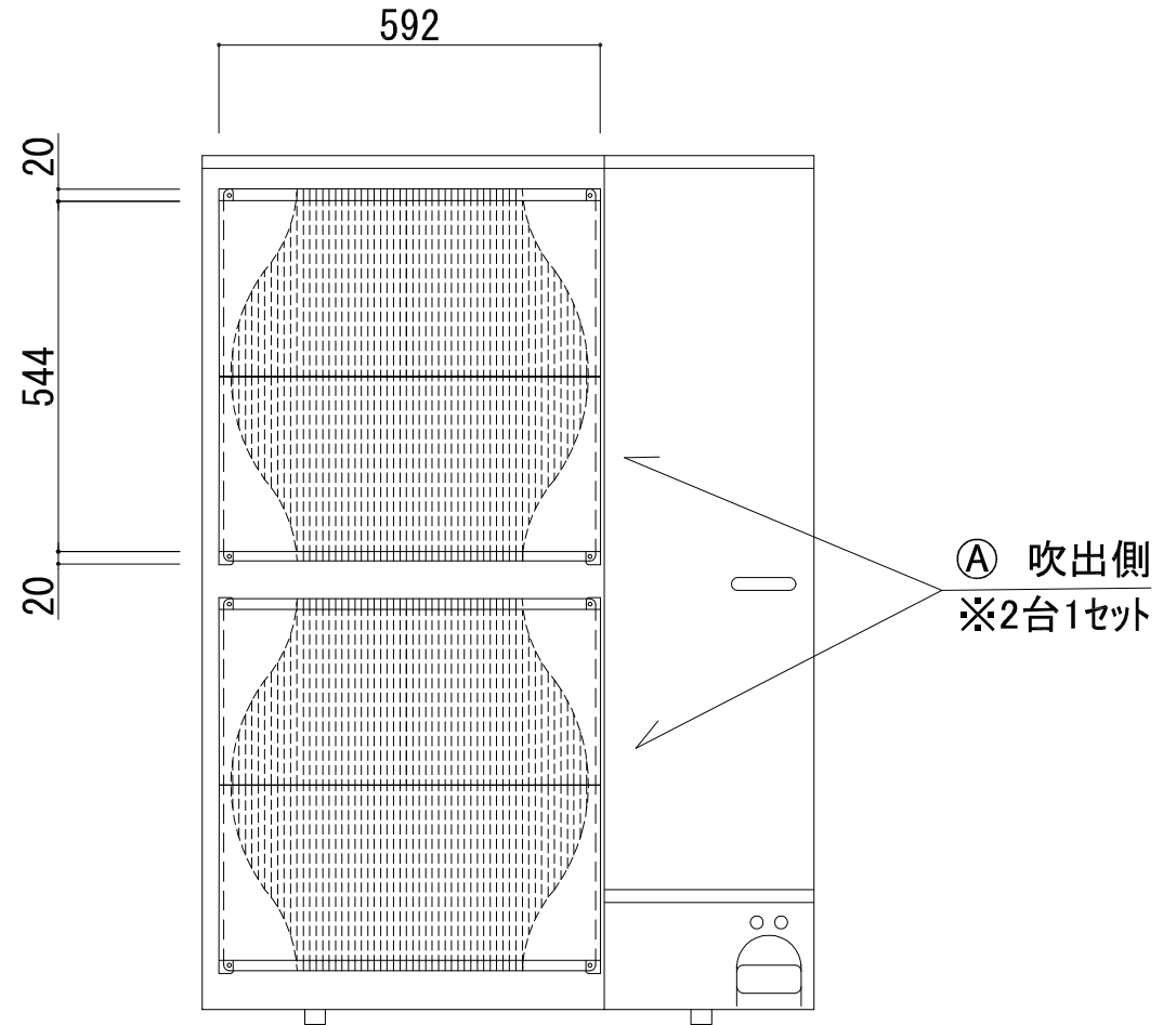
正面図
