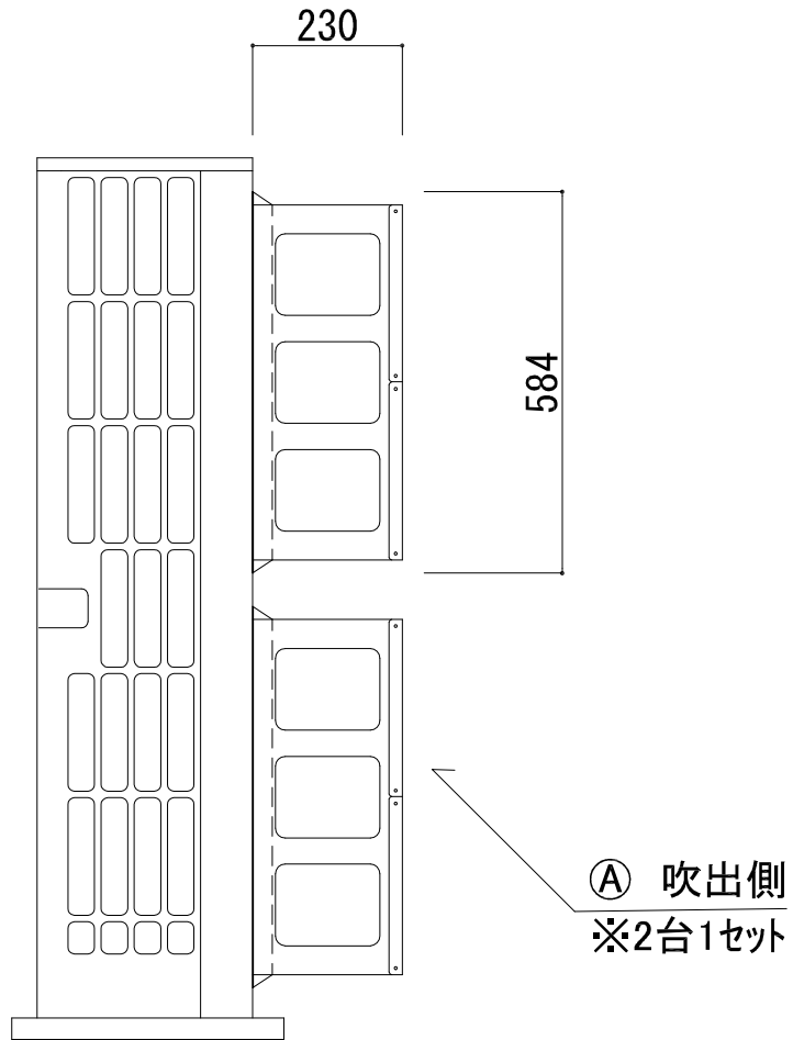
側面図
