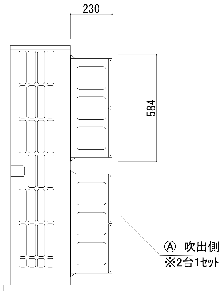
側面図
