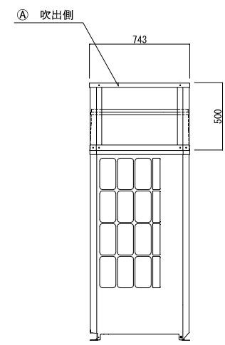
左側面図
