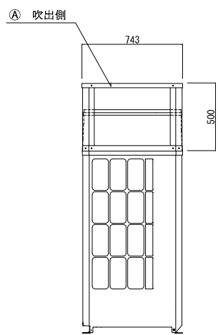
左側面図
