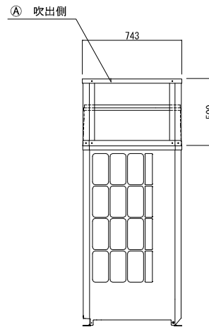
左側面図
