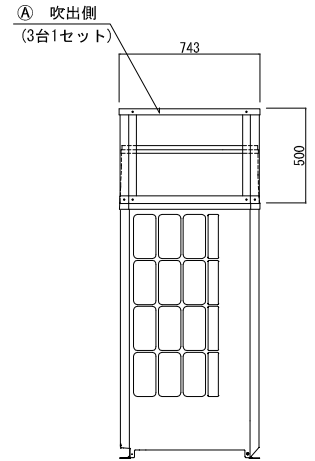
左側面図
