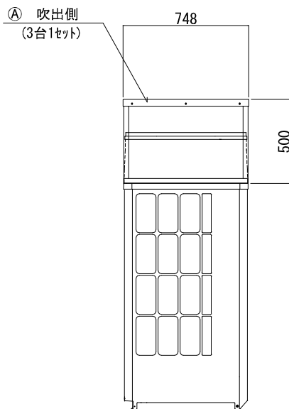
左側面図
