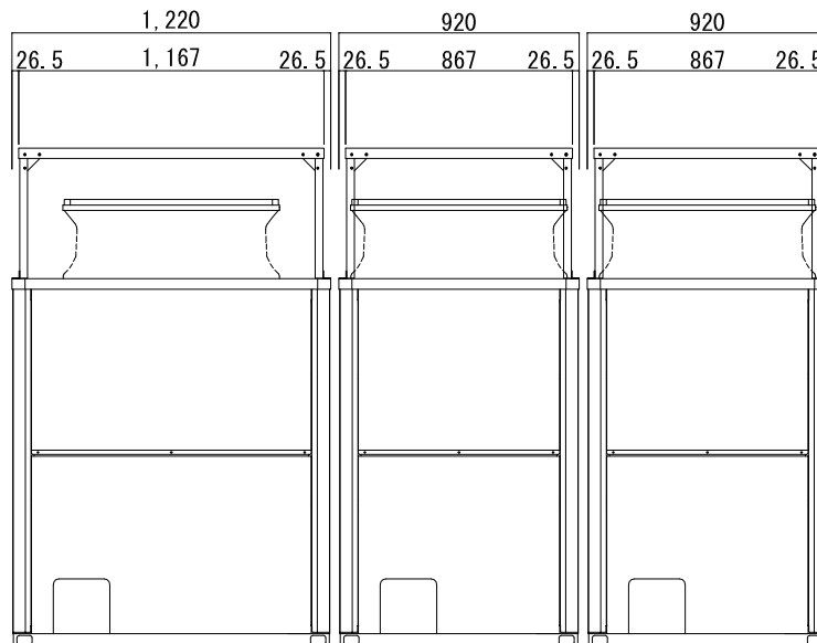
正面図
