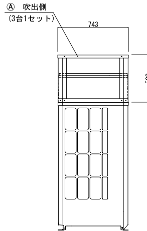
左側面図
