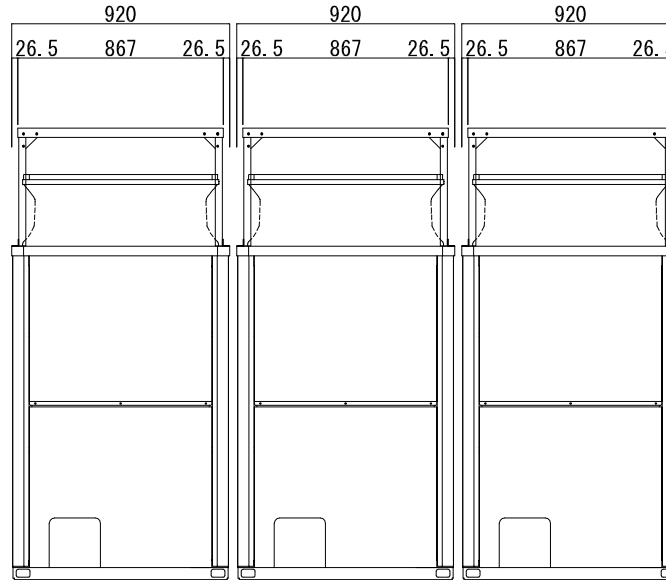
正面図
