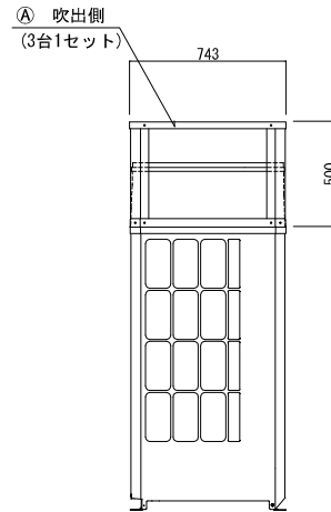
左側面図
