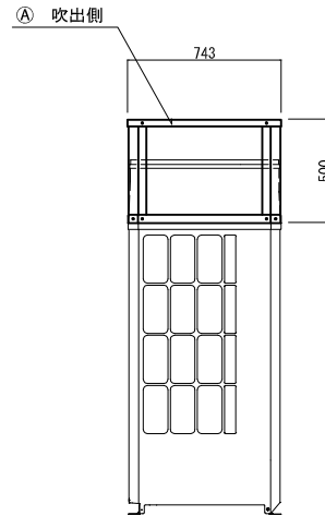
左側面図
