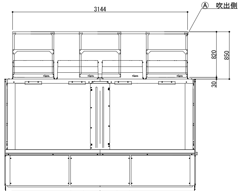
側面図
