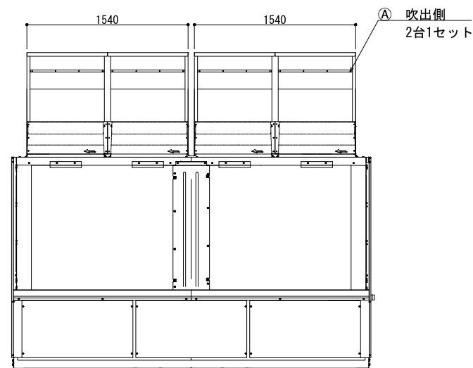
正面図
