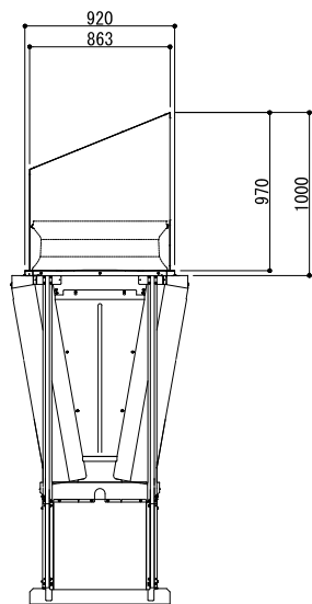
側面図
