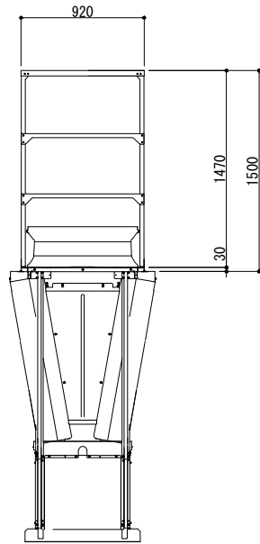
側面図
