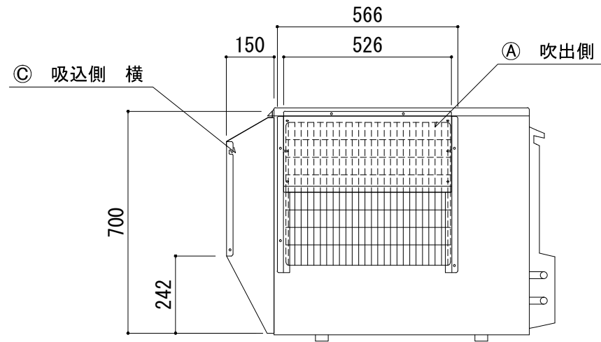
正面図
