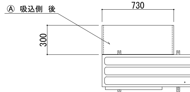
平面図
