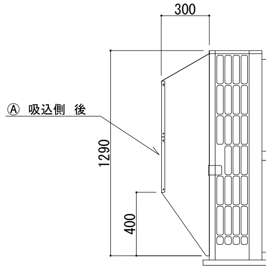
側面図
