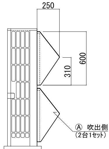
側面図
