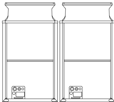
背面図
