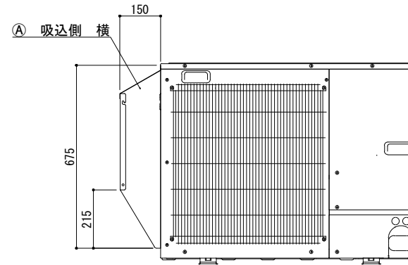
正面図
