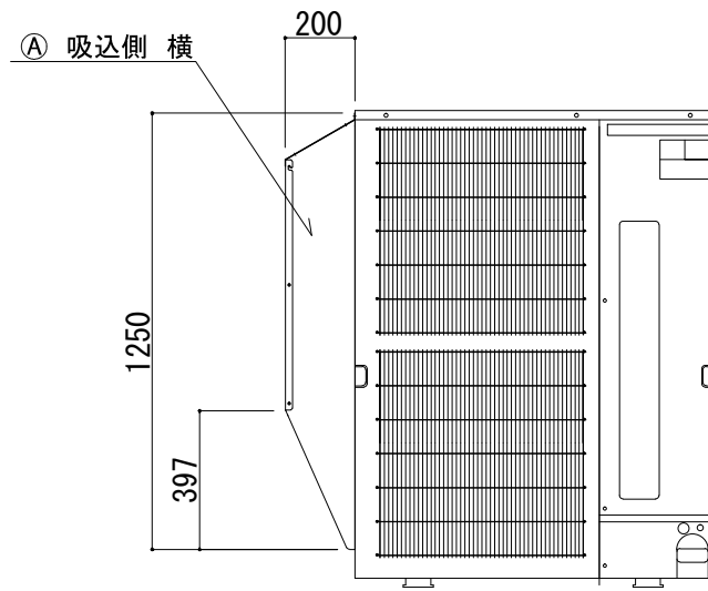
正面図
