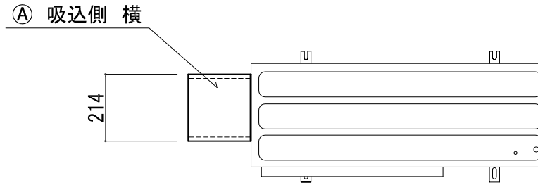
平面図
