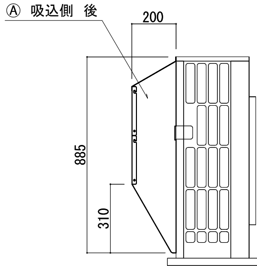
側面図
