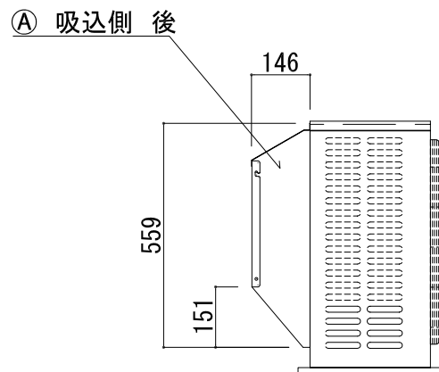
側面図
