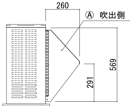
側面図
